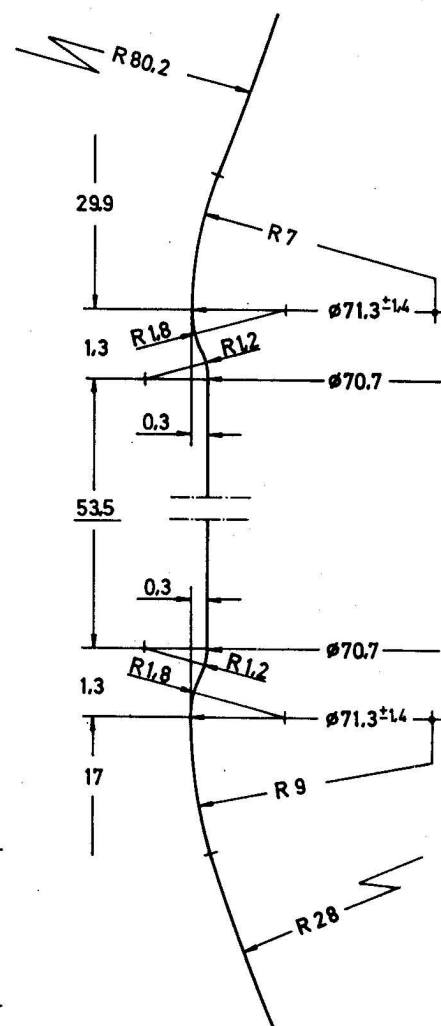
Detalle Z-Z
